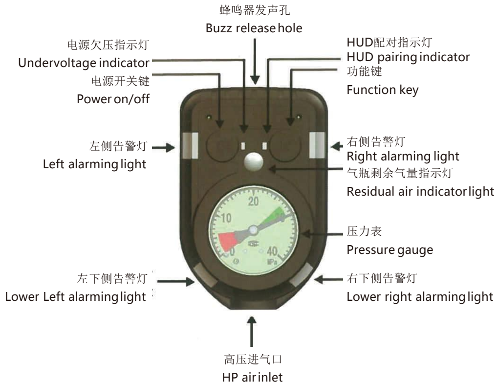
电子声光报警器 Electronic Audible and visual Alarm
